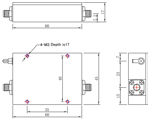
XB-07D UNIT:mm
